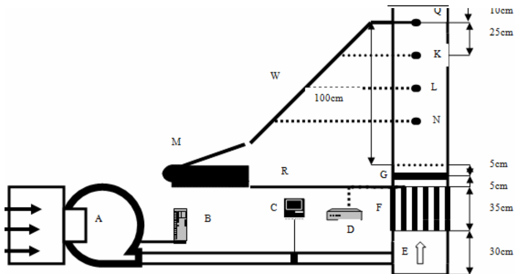
شکل ۲- شماتیک دستگاه اندازه‌گیری افت فشار. A فن و کانال ورودی، B مبدل ولتاژ، C سرعت سنج، D ترموستات، E ورودی هوا، F یکنواخت کننده هوا، G توری گالوانیزه، K، L، N و Q محل‌های سوراخ کاری شده، M مانومتر، W و R لوله‌های وصل شده به مانومتر
