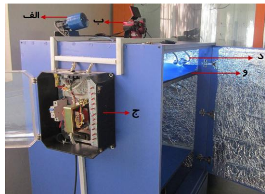
شکل ۳- اتاقک عکس برداری. الف) موتور، جهت تغییر ارتفاع صفحه ی پس زمینه. ب) دوربین که بر روی پایه ی اتاقک نصب شده است. ج) تابلوی کنترل روشنایی و لامپ های LED و راه اندازی موتور بالابرنده. د) لامپ LED به همراه پایه. و) صفحه ی پس زمینه
