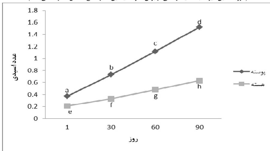
شکل ۳- نمودار تغییرات عدد اسیدی روغن پوسته و مغز هسته پسته گونه خینجوک
