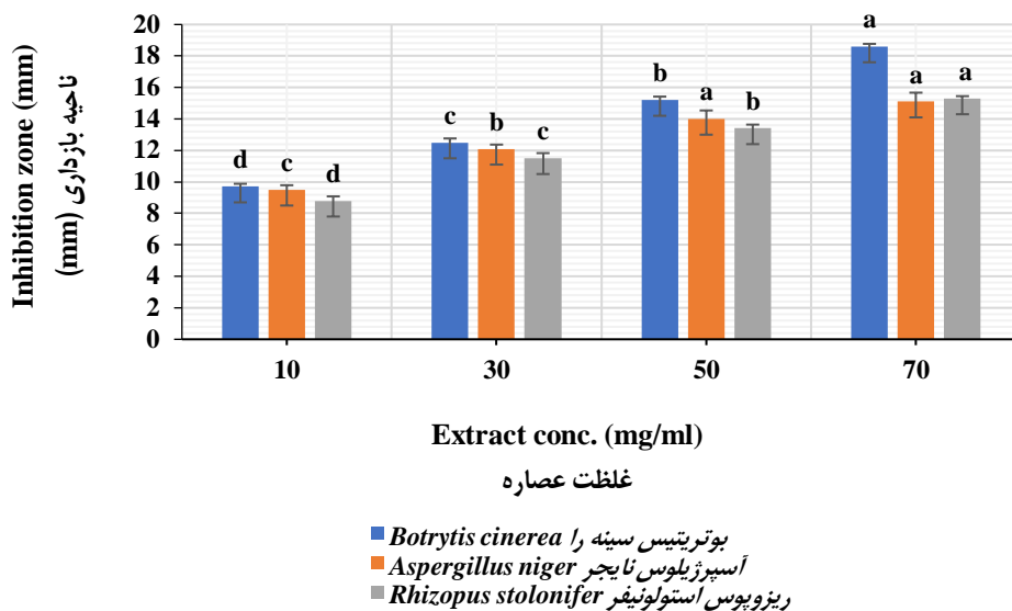
شکل ۴- فعالیت ضد قارچی عصاره اتانولی برگ چای سبز بر پایه روش چاهک آگار
