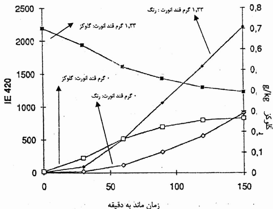
شکل ۹ - ارتباط خطی بین تشکیل رنگ و زمان ماند با توجه به مقدار قند انورت اولیه.
