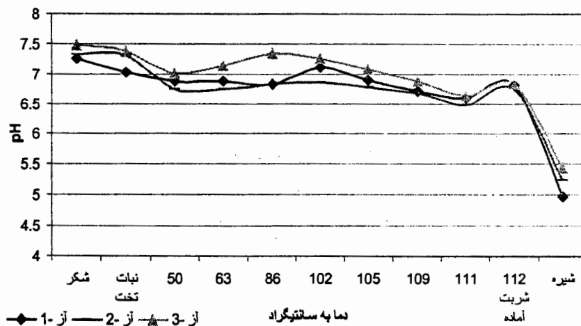
شکل ۱۱ - تغییرات pH طی حرارت دادن شربت.
