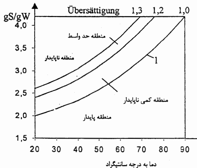
شکل ۴ - نسبت حلالیت ساکارز در آب و تغییرات میزان اشباعیت با توجه به درجه حرارت.
