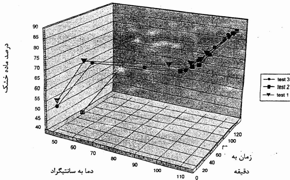
شکل ۷- تغییرات ماده خشک شربت در طی زمان آماده سازی شربت.
