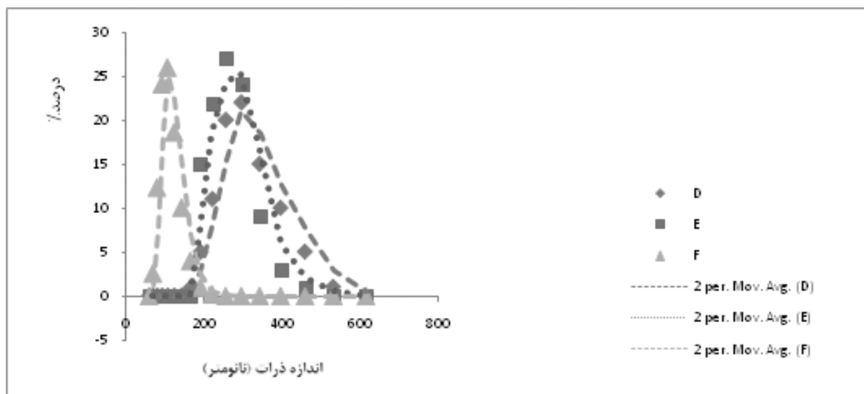
شکل ۱- منحنی توزیع اندازه قطرات امولسیون (D=۱%، E=۲۰%، F=۳۰% دیواره)
