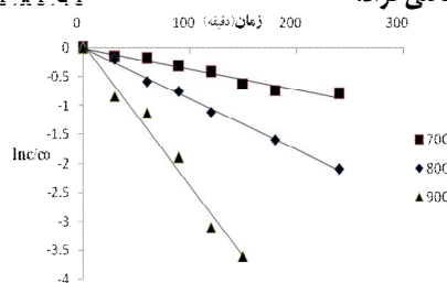
شکل ۴- تجزیه حرارتی آنتوسیانین‌های
