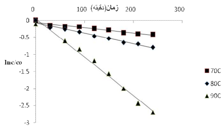
شکل ۳- تجزیه حرارتی آنتوسیانین‌های کنسانتره زرشک ( Bx=30 ) در دماهای
