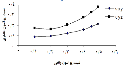
شکل ۳- رابطه‌ی بین نسبت پوآسون واقعی و ظاهری محاسبه شده‌ی مدل در دو امتداد xy و yz
