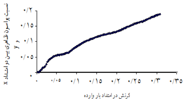
شکل ۴- نمونه‌ای از رابطه‌ی بین نسبت پوآسون ظاهری محاسبه شده‌ی مدل در امتداد xy با کرنش محوری در امتداد بار وارده (y) به ازاء مدول الاستیسیته‌ی ۱ مگاپاسکال و ضریب پوآسون واقعی ۰/۴۵
