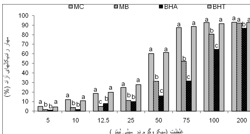
شکل ۱- مقایسه میانگین درصد مهار رادیکال‌های آزاد DPPH غلظت‌های مختلف عصاره‌های متانولی میوه‌ی دو وارپته بلوط و آنتی‌اکسیدان‌های سنتزی.
