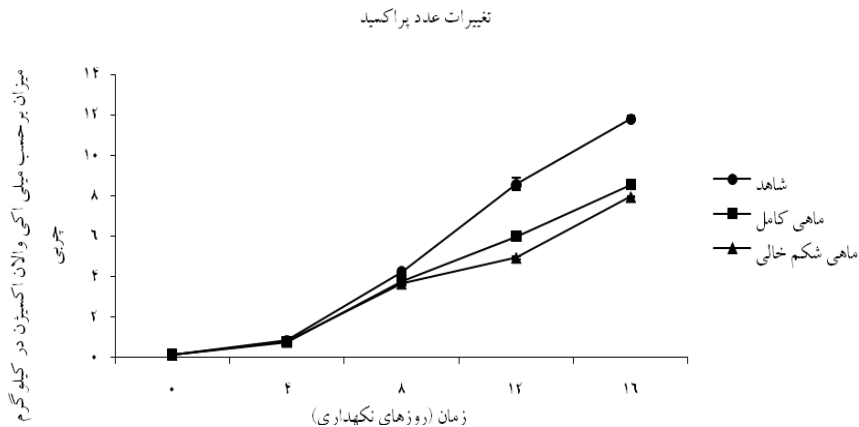
شکل ۱- تغییرات مقادیر عدد پراکسید (PV) برای تیمارهای مختلف آنتی‌کسیدان نسبت به زمان طی ۱۶ روز نگهداری در یخ
